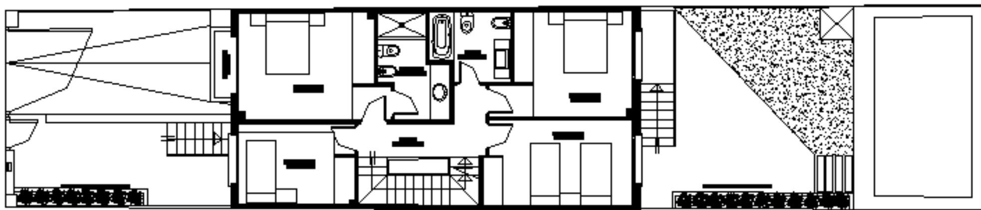
PLANTA PRIMERA
